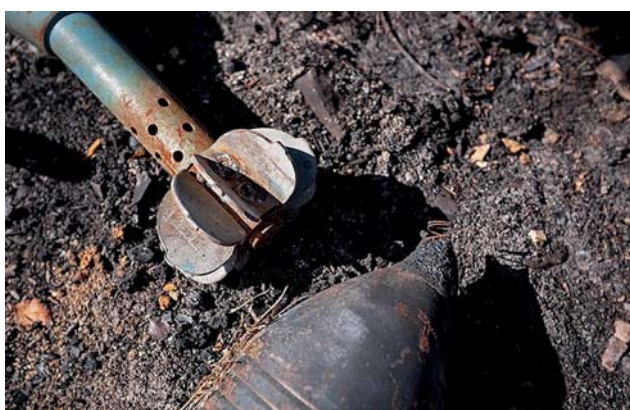
Рис. 5. Приваренные к корпусу мины элементы хвостового оперения
